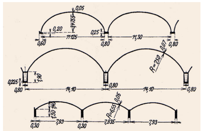
Bild 7 Entwicklung der Querschnitte der Tonnenschalen (von oben nach unten): Dywidaghalle auf der Gesolei 1 mit senkrechten Endtangente, Großmarkthalle Frankfurt a. M. mit Kreissegmentquerschnitt, Flugzeughalle Kowno (Kaunas, Litauen) Development of cross-sections for barrel vaults (top to bottom), Dywidaghalle with vertical edge tangents at the „Gesolei“ 2 , Central Market Hall in Frankfurt a. M. with circular segment cross-section, Airplane Hall in Kovno (Kaunas, Lithuania)
