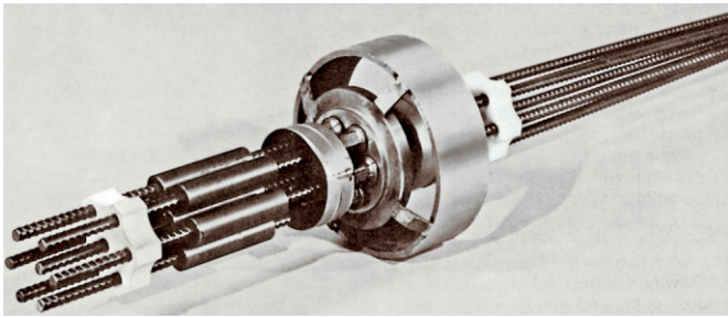
Bild 15 Glockenverankerung und Muffenstoß Bell anchorage and coupling edge
